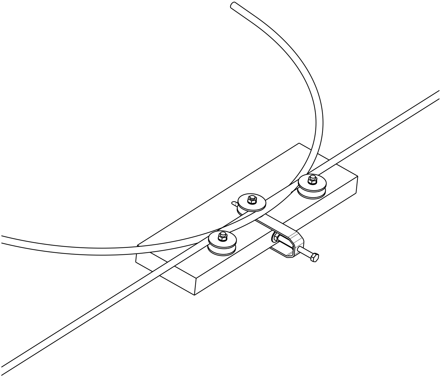
Isometric view Scale: 1:4
