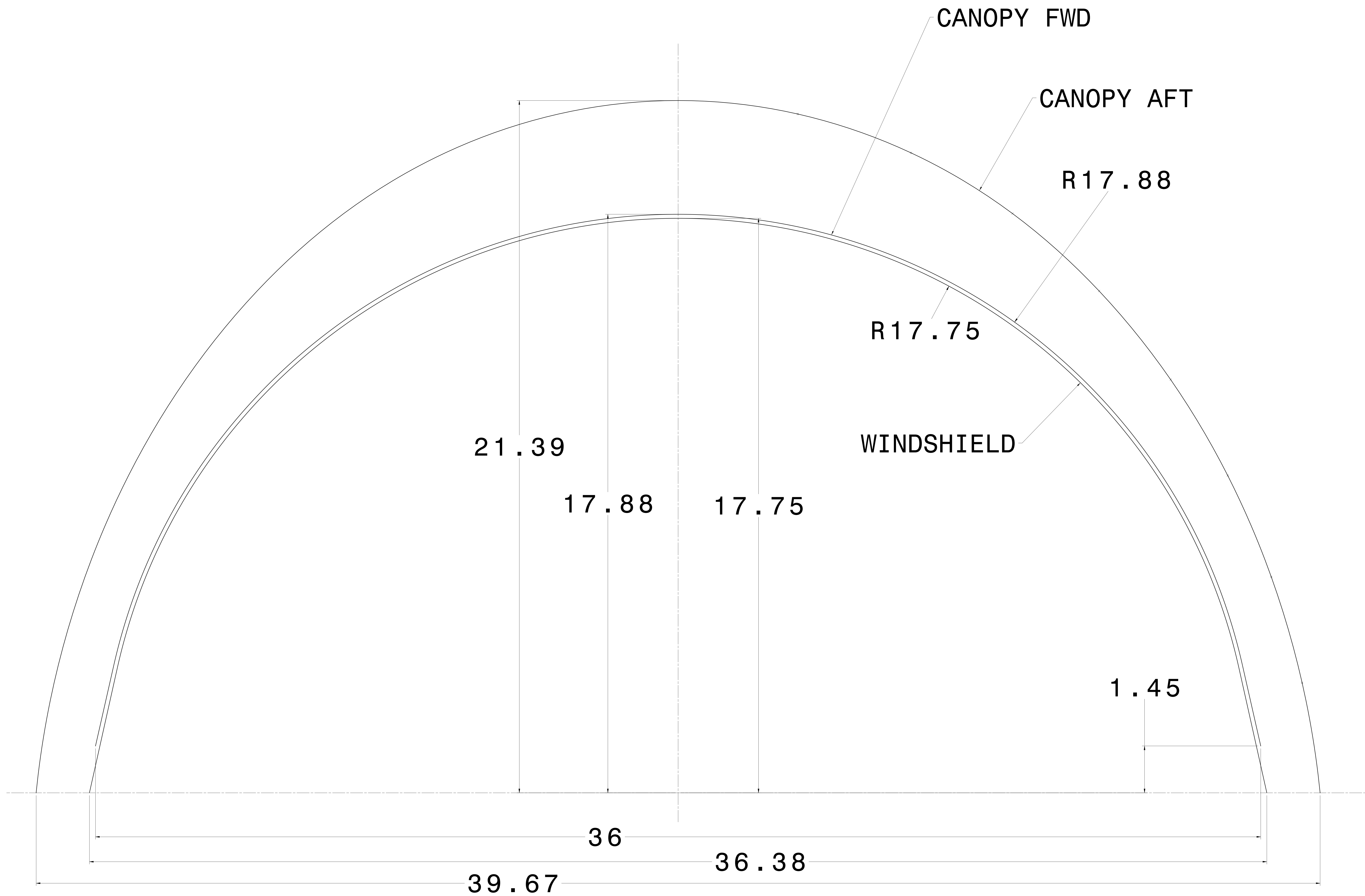
Front view Scale: 1:1
