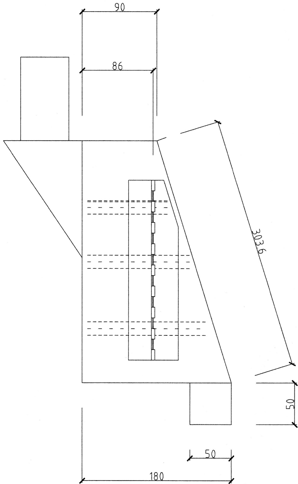
end elevation
